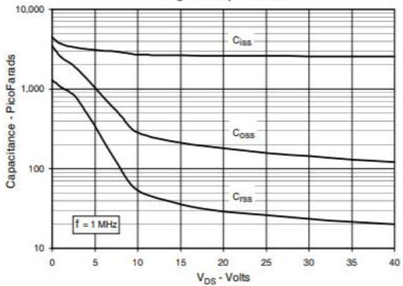
Fig. 11. Capacitance
