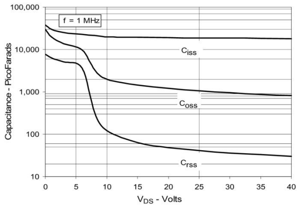
Fig. 11. Capacitance
