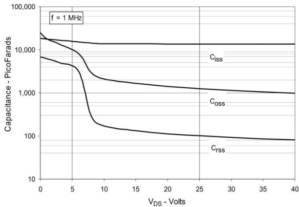
Fig. 11. Capacitance
